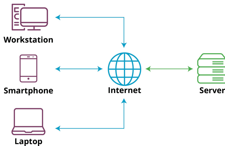
Slika 3.1 - Klijent-poslužitelj arhitektura [18]
