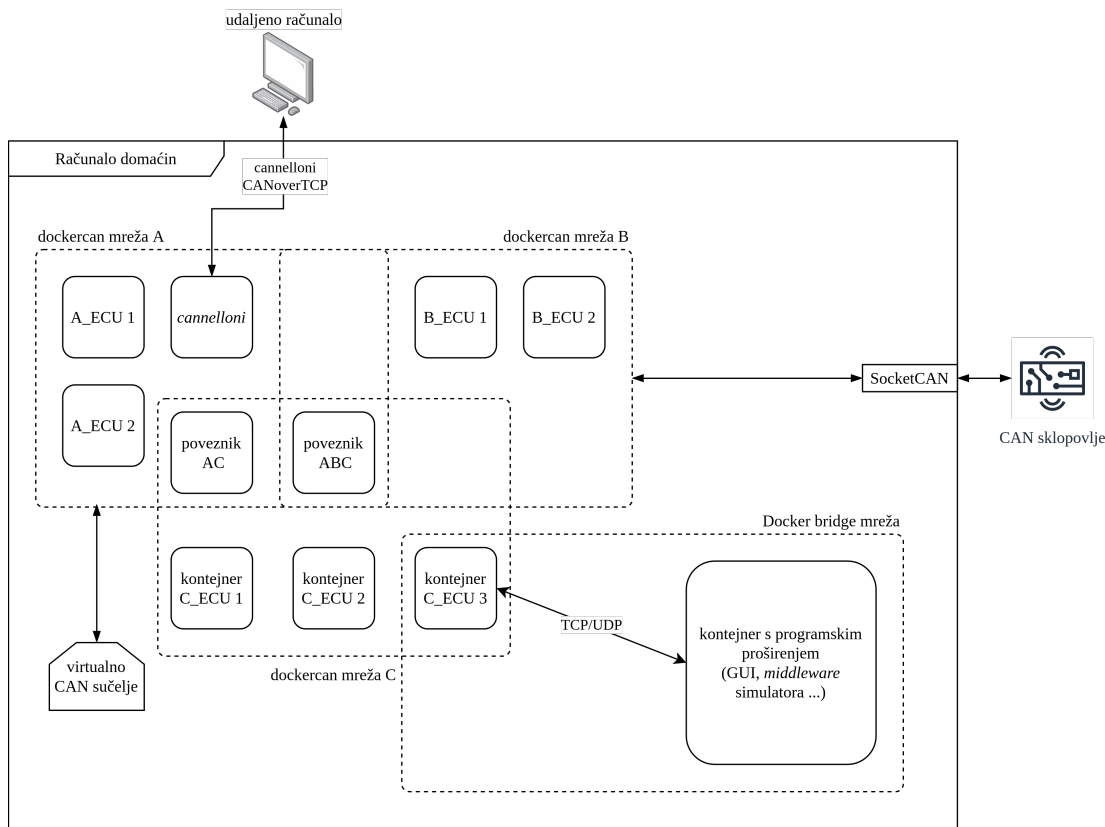
Slika 5.1: Arhitektura sustava
