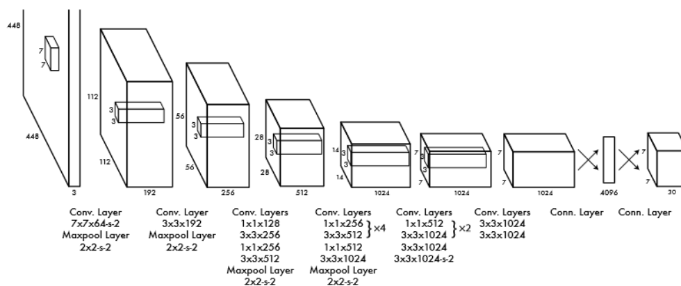
Slika 2.14. Arhitektura YOLO neuronske mreže (Redmon, 2016)
