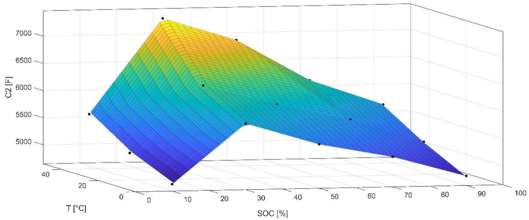
Sl. 3.11 Ovisnost parametra C_2 o SOC-u i temperaturi u troosnom prikazu
