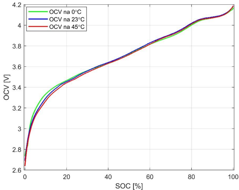
Sl. 1.1 OCV baterije pri različitom SOC-u i temperaturi
