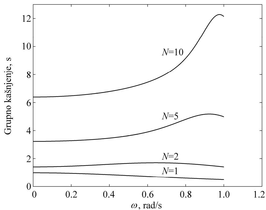
Slika 3.11 Grupno kašnjenje odziva na sinc puls Butterworthovog filtra od prvog do desetog reda granične frekvencije \omega_g = \omega_{3dB} = 1 \text{ rad/s} .
