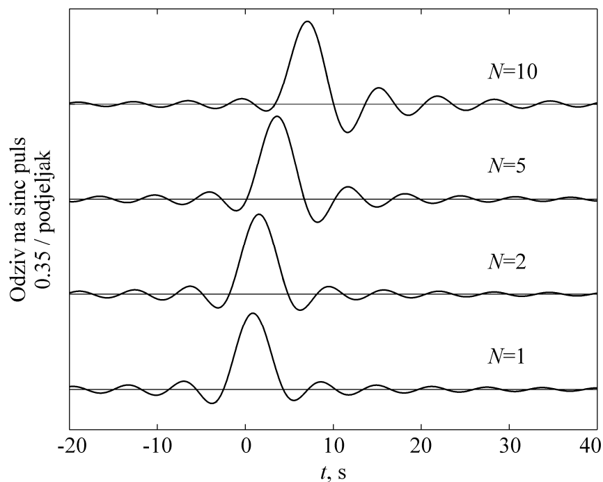
Slika 3.9 Odziv na sinc puls Butterworthovog filtera od prvog do desetog reda granične frekvencije \omega_g = \omega_{3dB} = 1\text{rad/s} .
