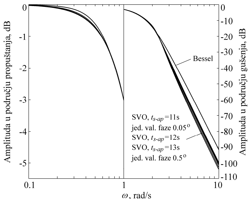
Slika 4.16 Amplitudna karakteristika niskopropusnih filtara šestog reda sa simetričnim vremenskim odzivom (SVO), Besselovog filtra i filtara s jednolikom valovitošću fazne pogreške od 0.5^\circ i 0.05^\circ , normirani na \omega_{3\text{dB}}=1\text{rad/s} .
