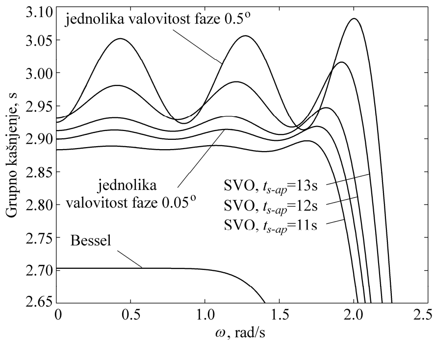
Slika 4.15 Grupno kašnjenje niskopropusnih filtara šestog reda sa simetričnim vremenskim odzivom (SVO), Besselovog filtra i filtara s jednolikom valovitošću fazne pogreške od 0.5^\circ i 0.05^\circ , normirani na \omega_{3\text{dB}}=1\text{rad/s} .
