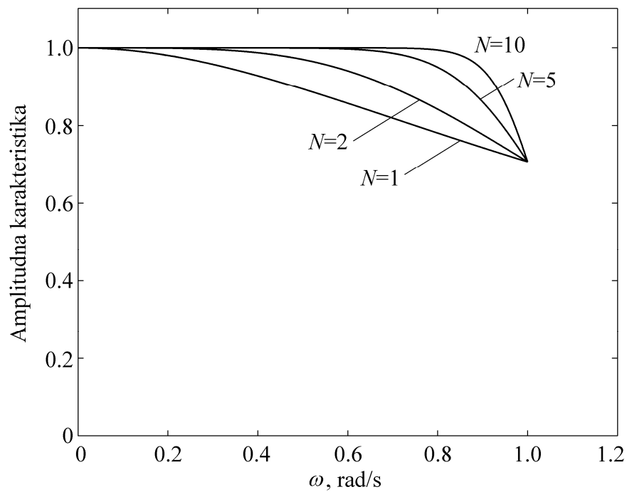
Slika 3.10 Amplitudna karakteristika odziva na sinc puls Butterworthovog filtra od prvog do desetog reda granične frekvencije \omega_g = \omega_{3dB} = 1 \text{ rad/s} .
