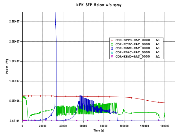
Slika 33: Distribucija snage (bez spreja, 10 cm 2 otvor)
