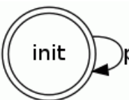
Slika 3.33: Büchijev automat za LTL formulu \square p
