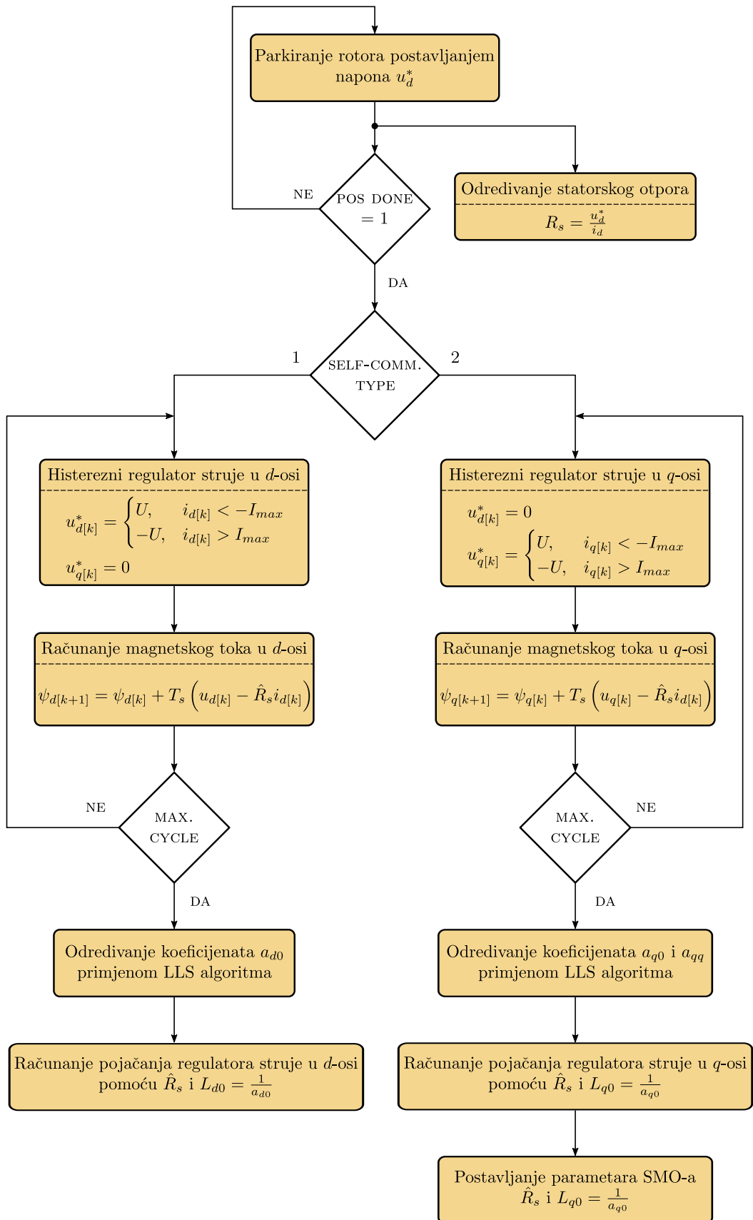
Slika 7.4: Dijagram toka za odredivanje statorskog otpora i koeficijenta a_{d0} , a_{q0} i a_{qq}
