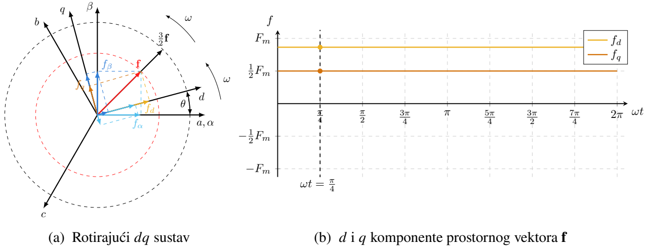
Slika 2.13: Parkova transformacija
