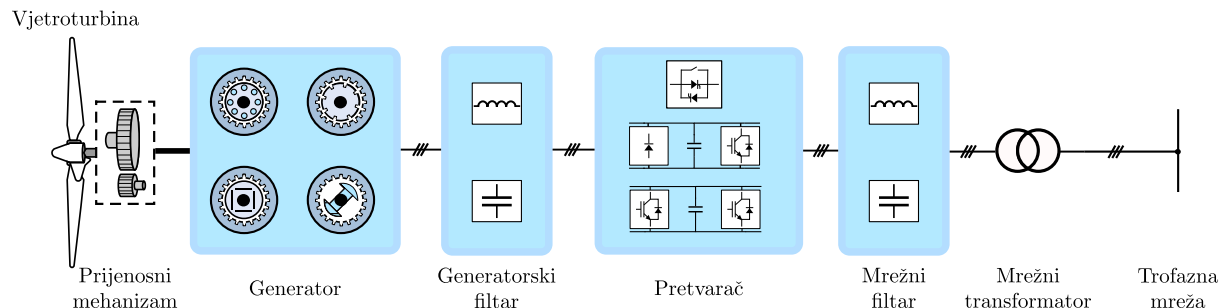
Slika 2.1: Općenita struktura sustava za pretvorbu energije vjetra
