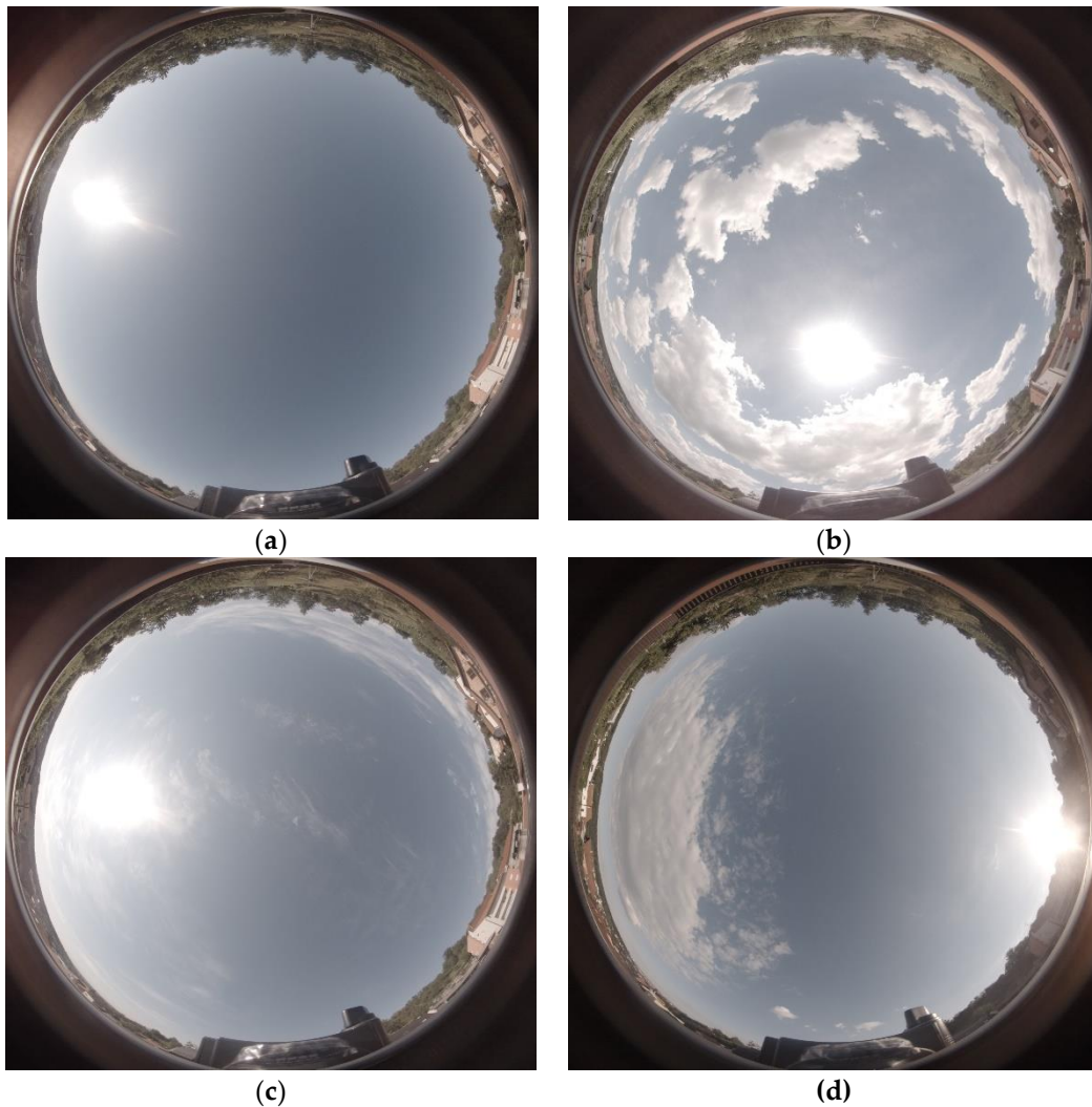
Slika 3.1: Primjeri slika neba: (a) slika čistog neba samo sa Suncem i bez oblaka snimljeno 13.07.2020. u 08:09:09, (b) slika sa Suncem i kumulacnim oblacima snimljena 13.07.2020. u 13:26:20, (c) slika sa Suncem i cirus oblacima snimljena 14.07.2020. u 09:09:15 te (d) slika snimljena krajem dana prije zalaska Sunca snimljena 14.07.2020. u 18:45:32.
