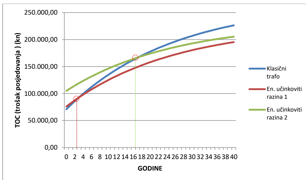
Slika 4-14 - Usporedba troška posjedovanja za slabo opterećeni transformator 630 kVA
