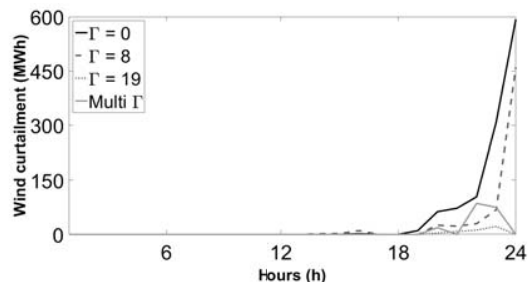
Fig. 3. Wind curtailment.
