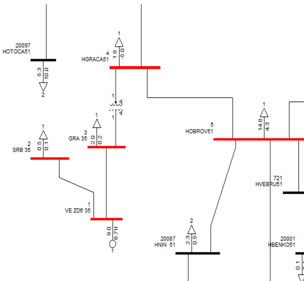
Slika 5.12 Ekranski prikaz proračuna tokova snaga u programskom paketu PSS/E za model vjetroelektrane Zadar 6
