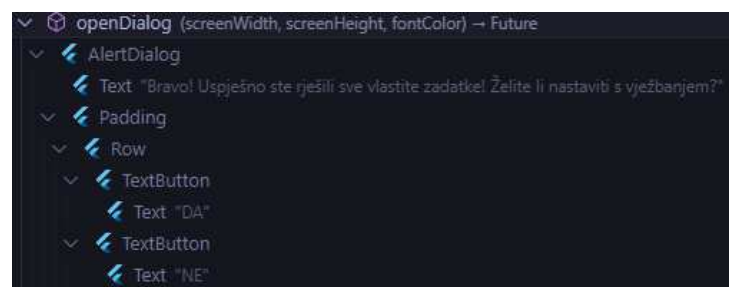
Slika 3.7 Stablo widgeta za funkciju koja otvara dijalog
