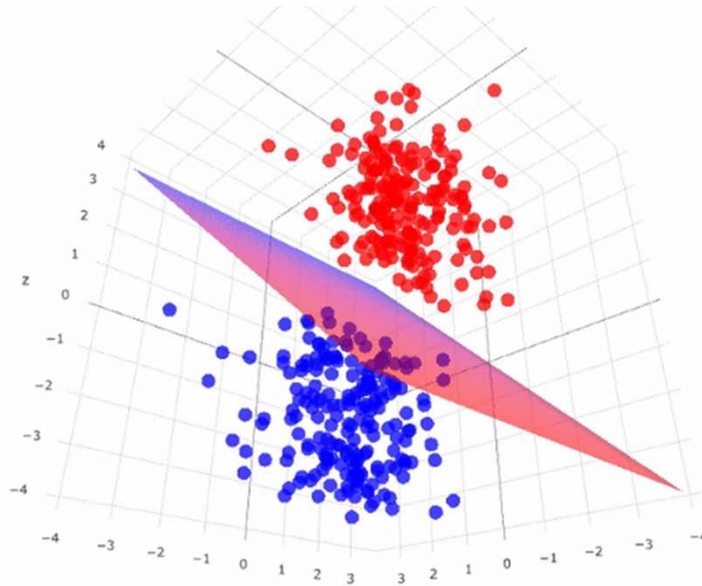
Slika 2.3. Stroj potpornih vektora na dvodimenzionalnom, linearno odvojuvom skupu podataka[4]
