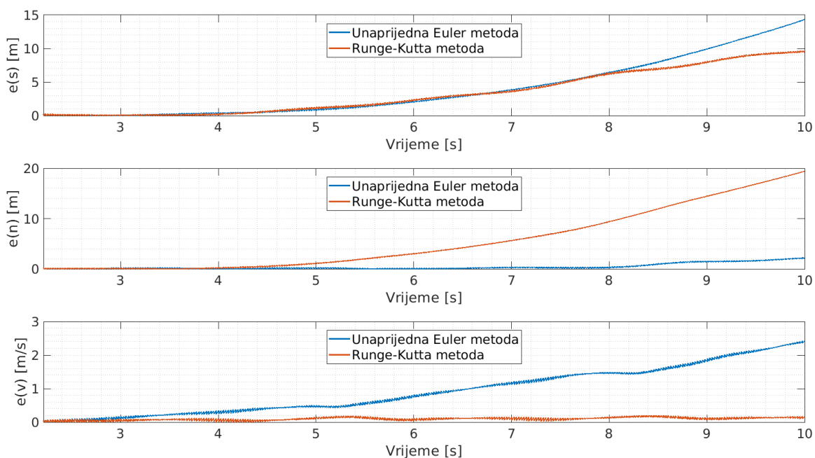
Slika 5.14. Greške predikcijskih modela.
