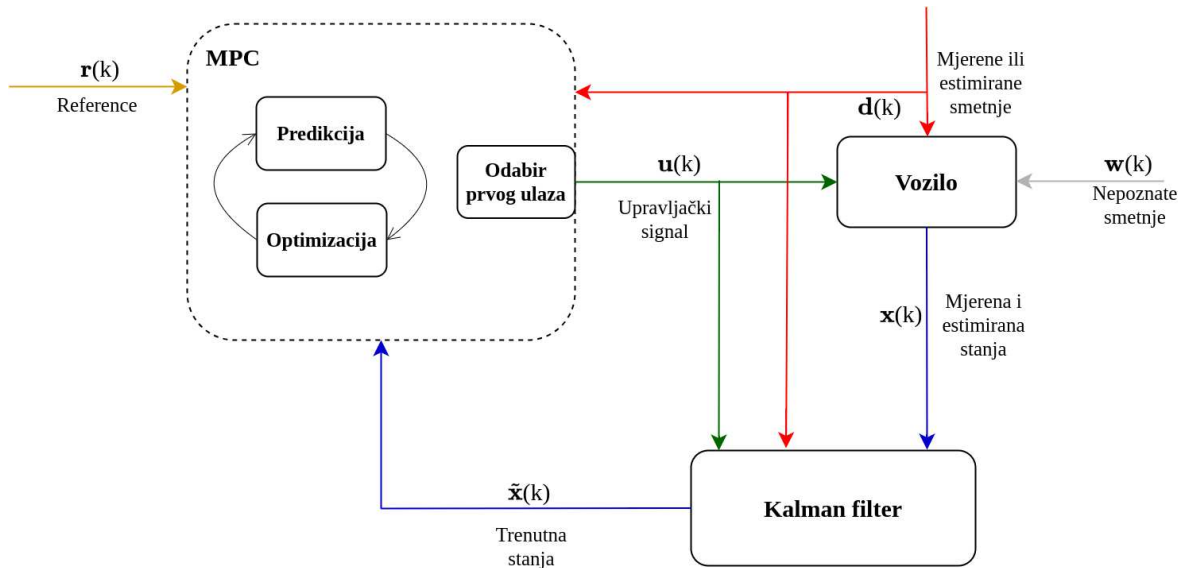
Slika 4.3. Modelsko prediktivno upravljanje u zatvorenoj petlji upravljanja.
