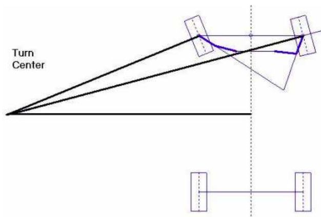
Slika 3.6. Ackermann geometrija skretanja.
