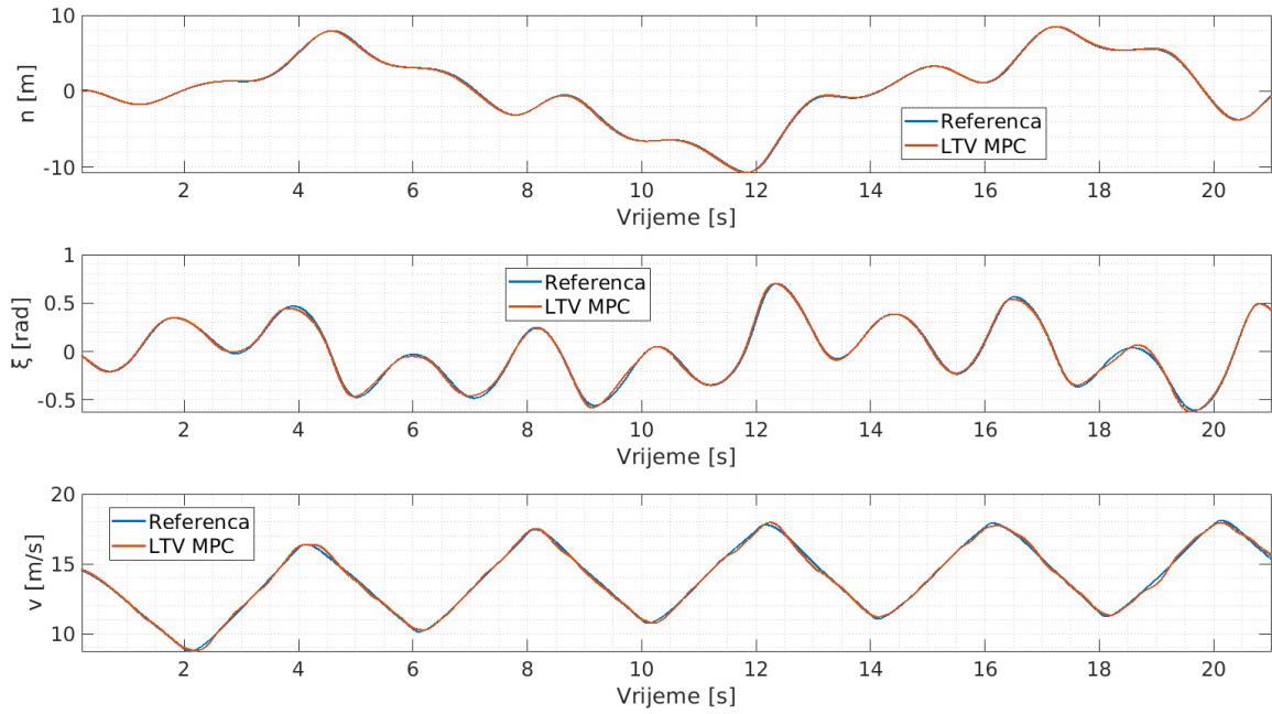
Slika 7.9. Praćenje reference varijabli stanja LTV MPC-a simulacije 6.
