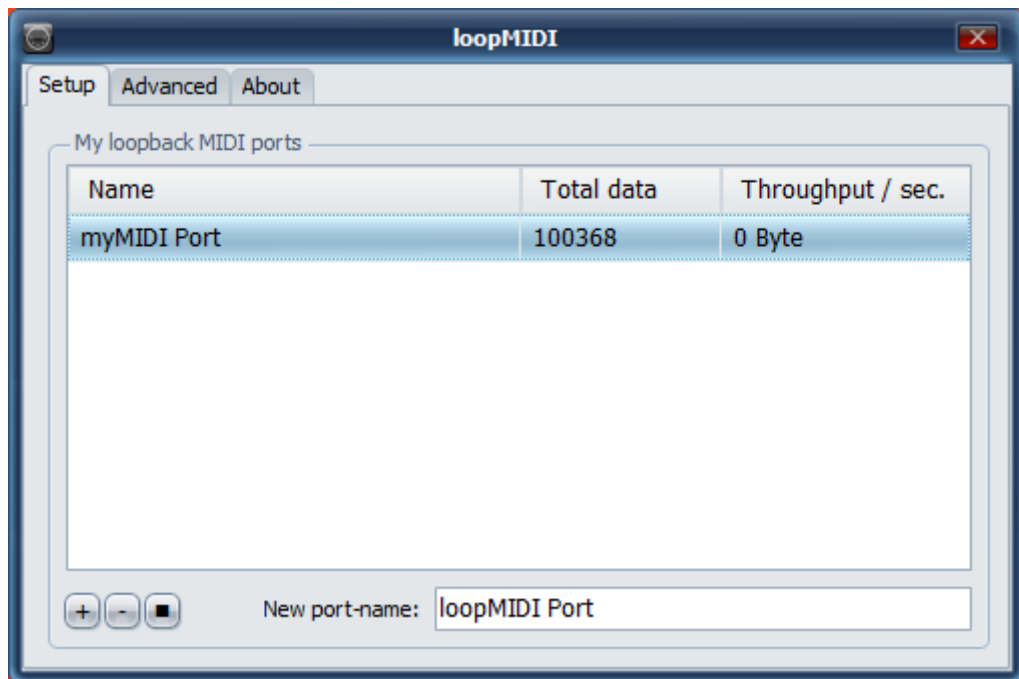
Slika 2.1 loopMidi
