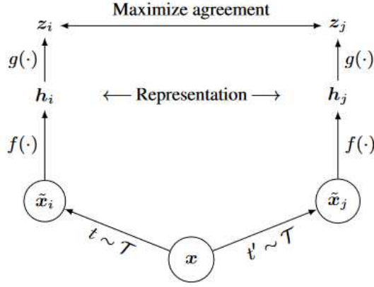
Slika 4.1: Prikaz SimCLR modela. Originalni primjer \mathbf{x} se deformira slučajnim deformacijama t i t' , na dobivene poglede \tilde{\mathbf{x}}_i i \tilde{\mathbf{x}}'_i primjenjuje se okosnica f(\cdot) . Izlazi iz okosnice, \mathbf{h}_i i \mathbf{h}'_i , su reprezentacije primjere, no pri učenju optimiramo razliku reprezentacija \mathbf{z}_i i \mathbf{z}'_i dobivene iz jednostavne projekcijske glave g(\cdot) . Slika preuzeta iz [5].
