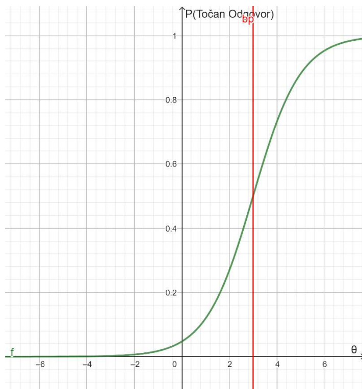
Slika 1 Utjecaj parametra b (težina zadatka) na logističku krivulju ( a = 1, c = 0, d = 1 ): b = 1 [gore] i b = 3 [dolje]
