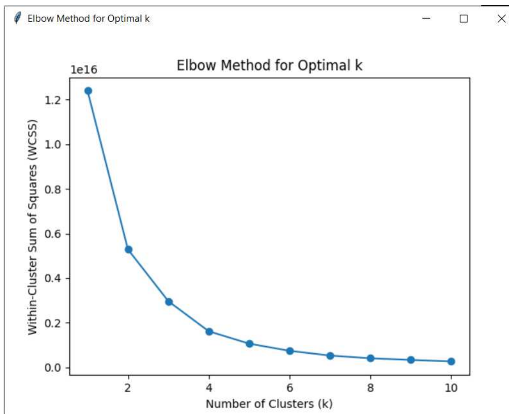
Slika 4.4 Elbow metoda na skupu automobila
