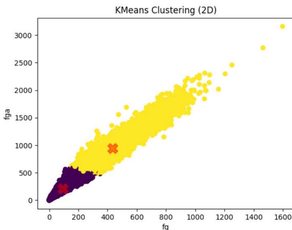
Slika 4.6 Grafički prikaz grupa košarkaša
