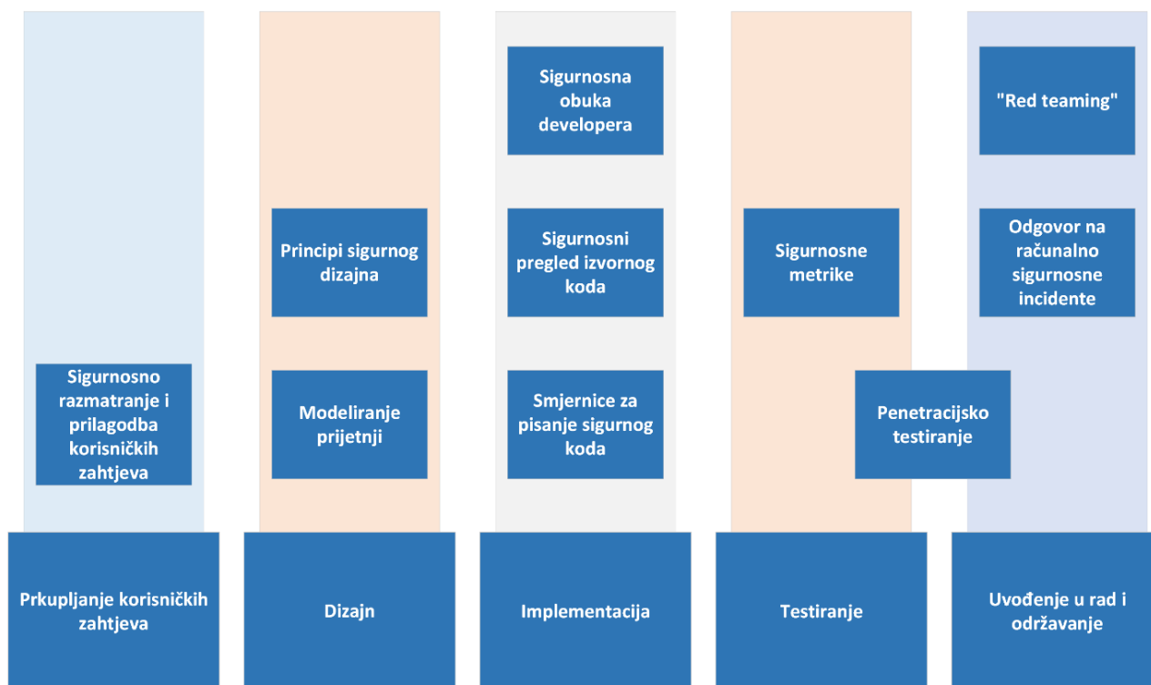
Slika 2.1. Model SSDLC procesa. Dijagram je temeljen na sintezi informacija iz različitih izvora, pri čemu su se primarno koristile informacije sadržane u sklopu sljedećeg online izvora: https://owasp.org/ .
