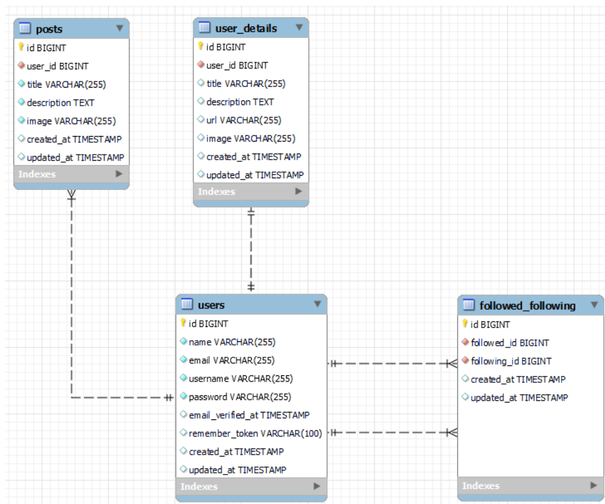
Slika 6.5. ER dijagram
