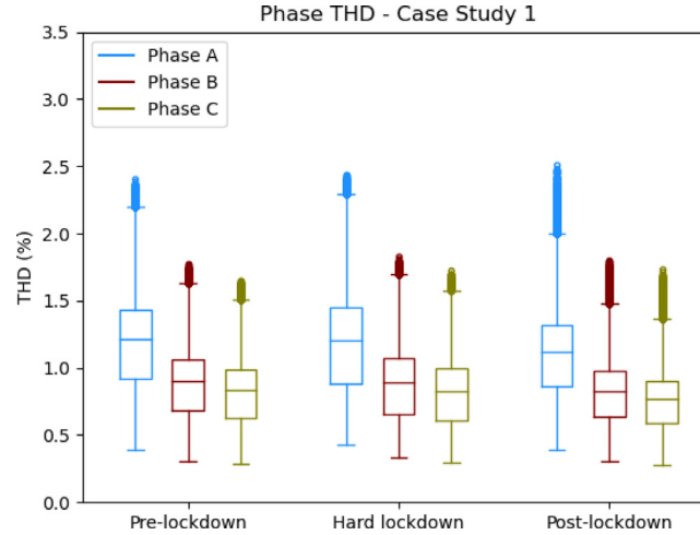
Fig. 6. THD (%) - CS1.
