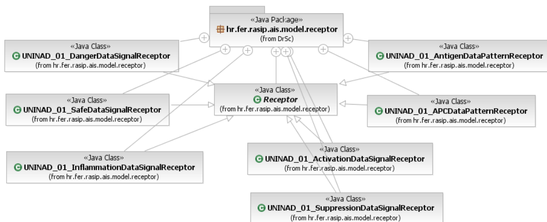
Slika 6.6 Dijagram razreda algoritma UNINAD paketa hr.fer.rasip.ais.model.receptor
