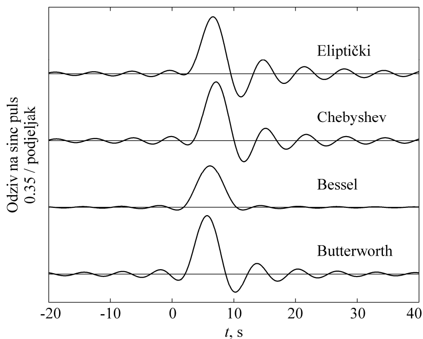
Slika 3.6 Odziv na sinc puls nekih klasičnih filtera osmog reda, svi normirani na \omega_g=1 rad/s.
