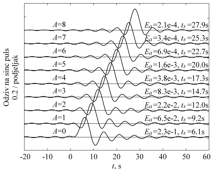
Slika 4.3 Odziv na sinc puls kaskade eliptičkog filtra osmog reda s 0.1dB valovitosti u području propuštanja, te 80dB valovitosti u području gušenja i optimalnog korektora A -tog reda, uz \omega_g = \omega_{0.1\text{dB}} = 1\text{rad/s} .
