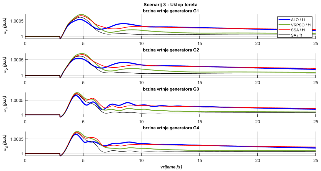
Slika 6.36. TAFM, scenarij 3 – odzivi brzina vrtnje generatora prema algoritmu i jednociljnoj metodi f_1(t) (4.2)
